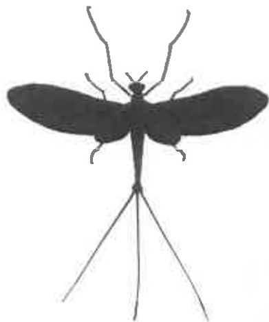
LEPTOPHLEBIA
